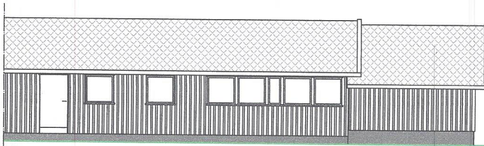
FASADE VEST
