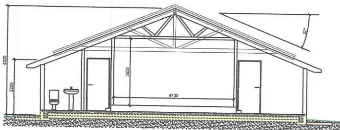
SNITT TILBYGG
