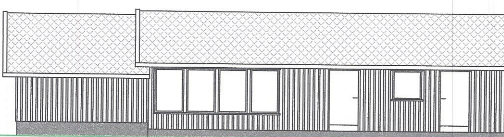
FASADE ØST
