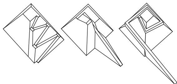
Différents types de rampes de construction.
